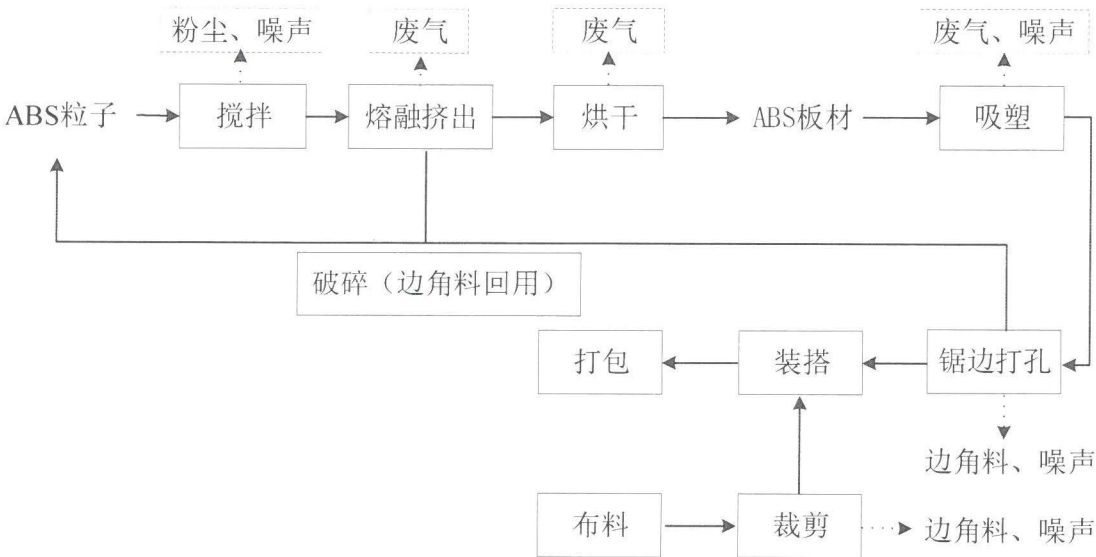
图 1 ABS 拉链箱包工艺流程图
