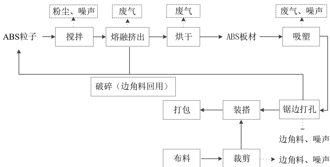
图 2.2.1-1 ABS 拉链箱包工艺流程图
