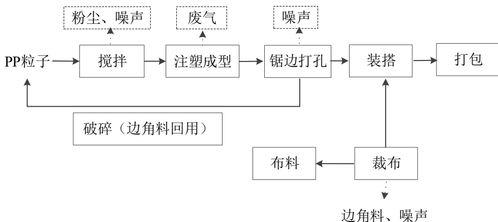
图 2.2.1-2 PP 箱包工艺流程图
